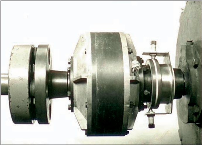
Az egyetemi első díjas TDK-munka a valóságban fékpadra szerelve (1975)
