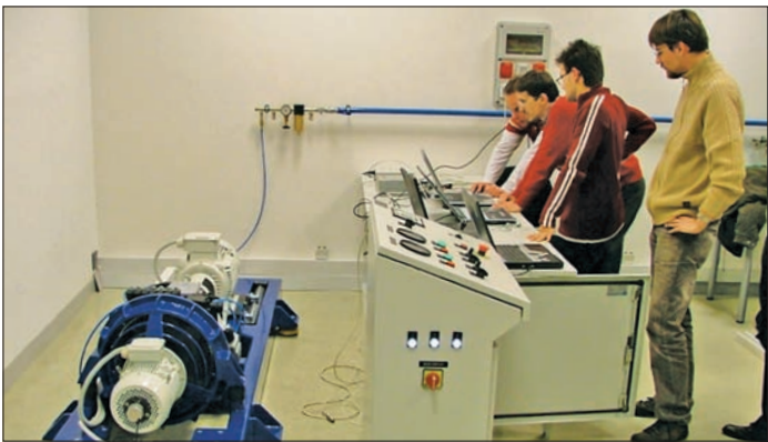
Sebességváltó tesztpad működés közben
