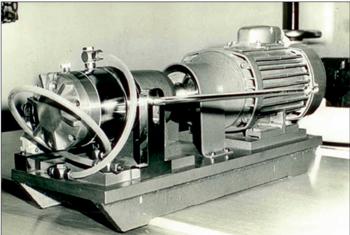
A doktori értekezés melléklete az írásztalon is elférő mágnesporos tesztpad (1978)
