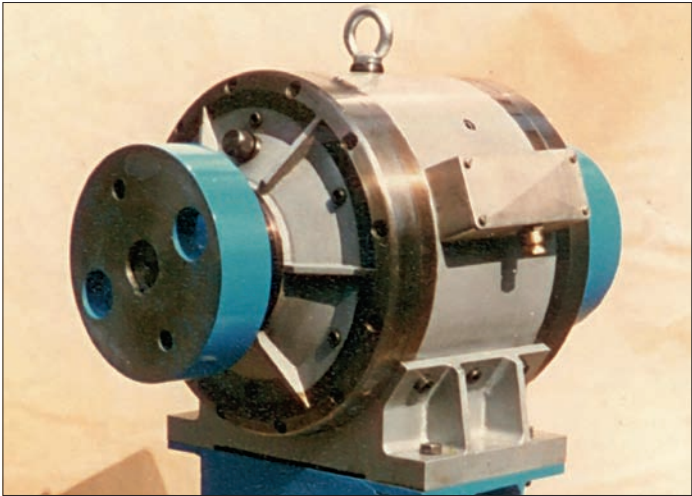
Az első bolygóműves automata sebességváltó, amelyet Simonyi Sándor tervei alapján az SVT-ben gyártottak le (1980)
