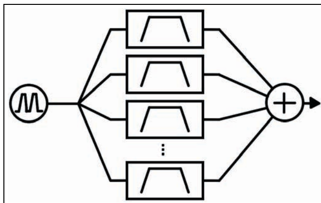
7.5. ábra. Ekvalizátorral megvalósított formáns szintézis blokkdiagramja.
