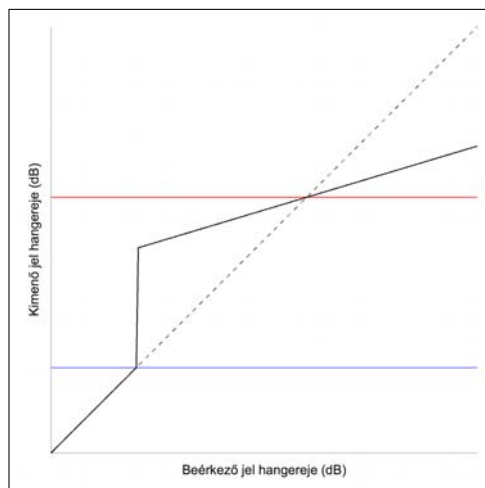
14.5. ábra. A HApp_14_01 (OSX) (WIN) programban alkalmazott tömörítő teljes karakterisztikája. A fekete vonal magát a karakterisztikát, a piros vonal a határértéket, a kék vonal pedig az aktiválódáshoz szükséges minimális hangerő szintjét mutatja.
