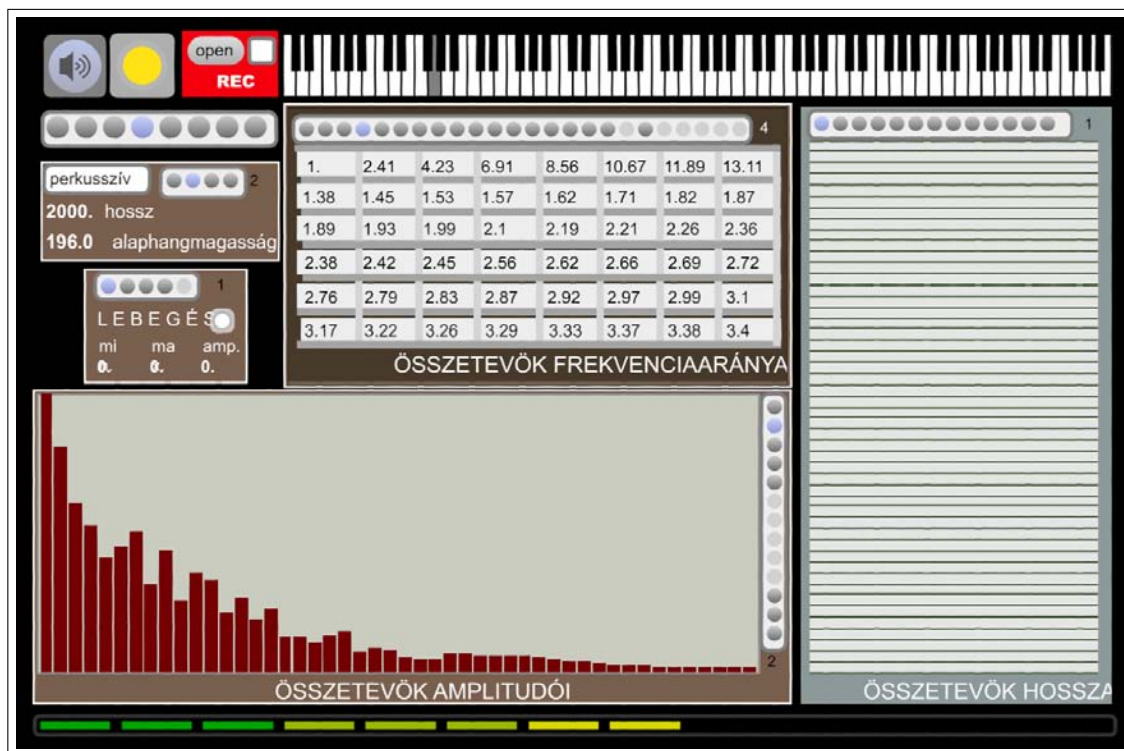
3.4. ábra. Negyvennyolc csatornás additív szintetizátor.
