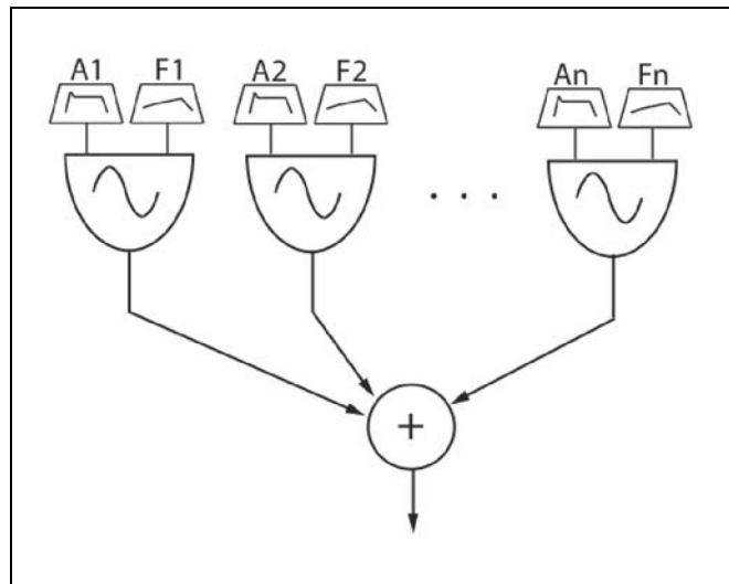
3.1. ábra. Additív szintetizátor sematikus modellje, ahol minden oszcillátor (időben változó) frekvenciája és amplitúdója egyedileg szabályozható.
