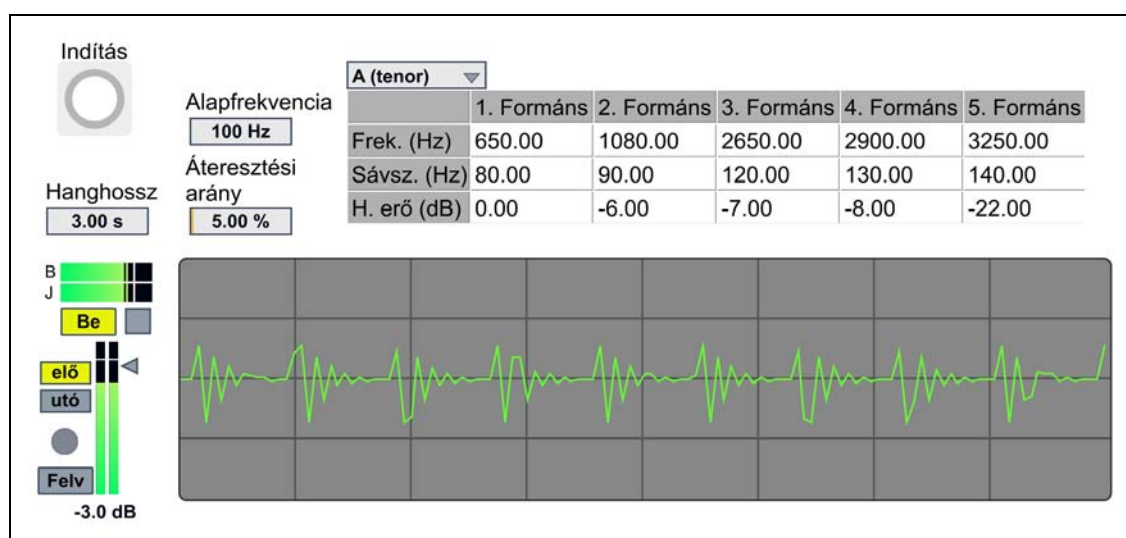
7.6. ábra. HApp_07_01 (OSX) (WIN): Formáns szintézis szűrőkkel.
