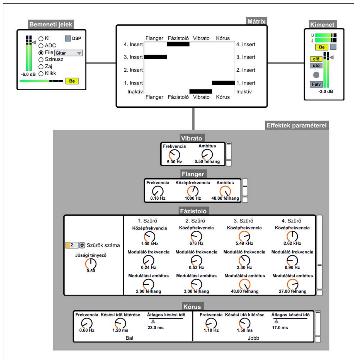
12.6. ábra. Késleltetésre/szűrésre épülő modulok Max programnyelven: Vibrato, Flanger, Fázistoló és Kórus.
