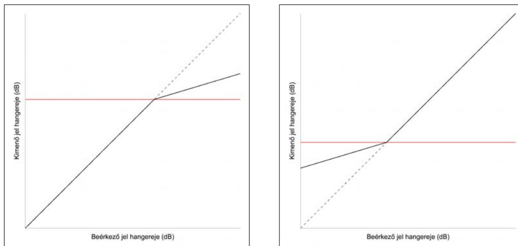
14.1. ábra. Egyszerű kompresszorok sematikus karakterisztikái. A piros vonalak mindkét ábrán az aktiválódás határértékét, a feketék a végső hangerő-karakterisztikát mutatják. A bal oldali ábra a határérték felett halkít, a jobb oldali a határérték alatt erősít. Mindkét esetben meggyelhető, hogy az eszköz egy nagyobb dinamika-tartományt képez le egy kisebbre.
