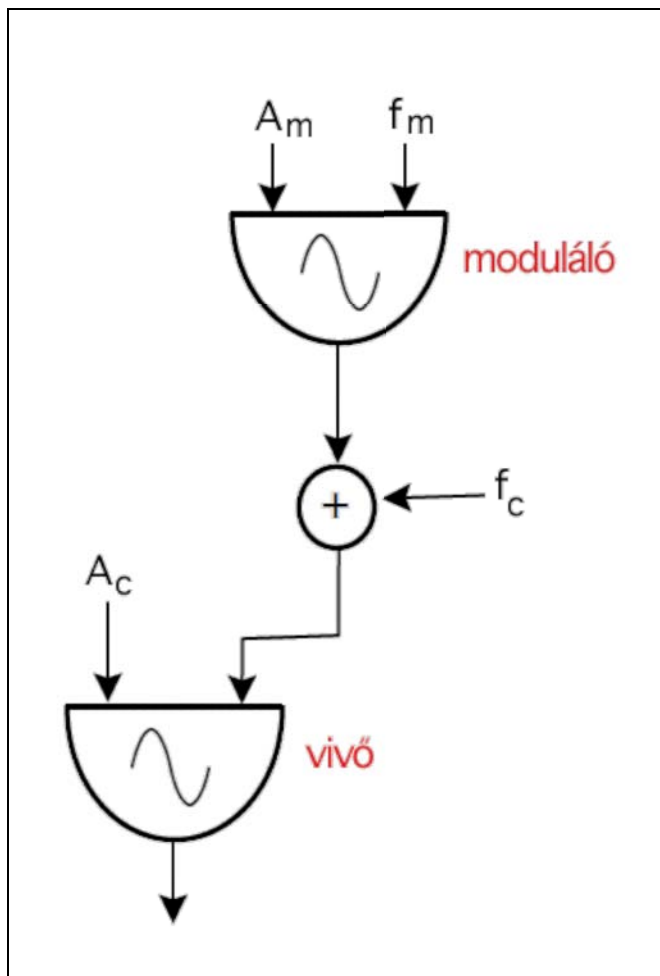
9.1. ábra. A frekvencia-moduláció folyamatábrája.
