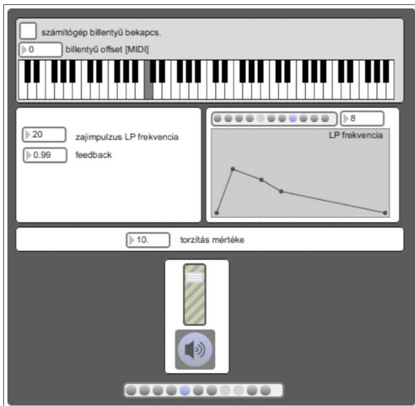
6.5. ábra. Karplus–Strong algoritmus Max programnyelven. A példát a HApp_06_01 (OSX) (WIN) program tartalmazza.
