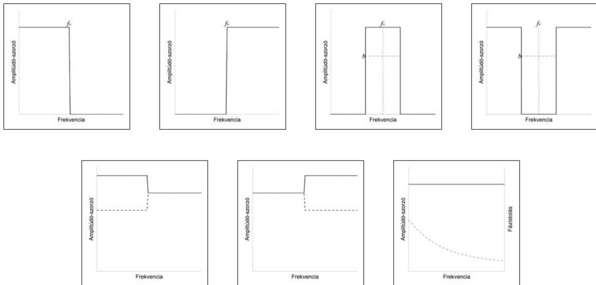
4.2. ábra. A legfontosabb szűrőtípusok idealizált amplitúdó-karakteristikái. Felső sor (balról jobbra): aluláteresztő, felüláteresztő, sáváteresztő, sávzáró; alsó sor (balról jobbra): low-shelf, high-shelf, mindent áteresztő. f_c (típustól függően) a levágási- vagy a középfrekvenciát, míg b a sáv szélességet jelöli. A valóságban a karakterisztikák levágása sosem végtelenül éles; a levágási tartomány meredeksége fontos jellemzője az adott szűrő minőségének. A mindent áteresztő szűrő esetén (mivel amplitúdó-karakterisztikája teljesen vízszintes) feltüntettük a fázis-karakterisztikát is.
