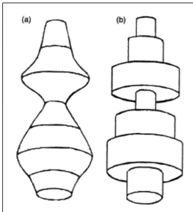
6.3. ábra. Egy szabálytalan cső közelítése hengeres hullámvezetőkkel: az eredeti, komplex cső (a) és a hullámvezető-modell (b).
