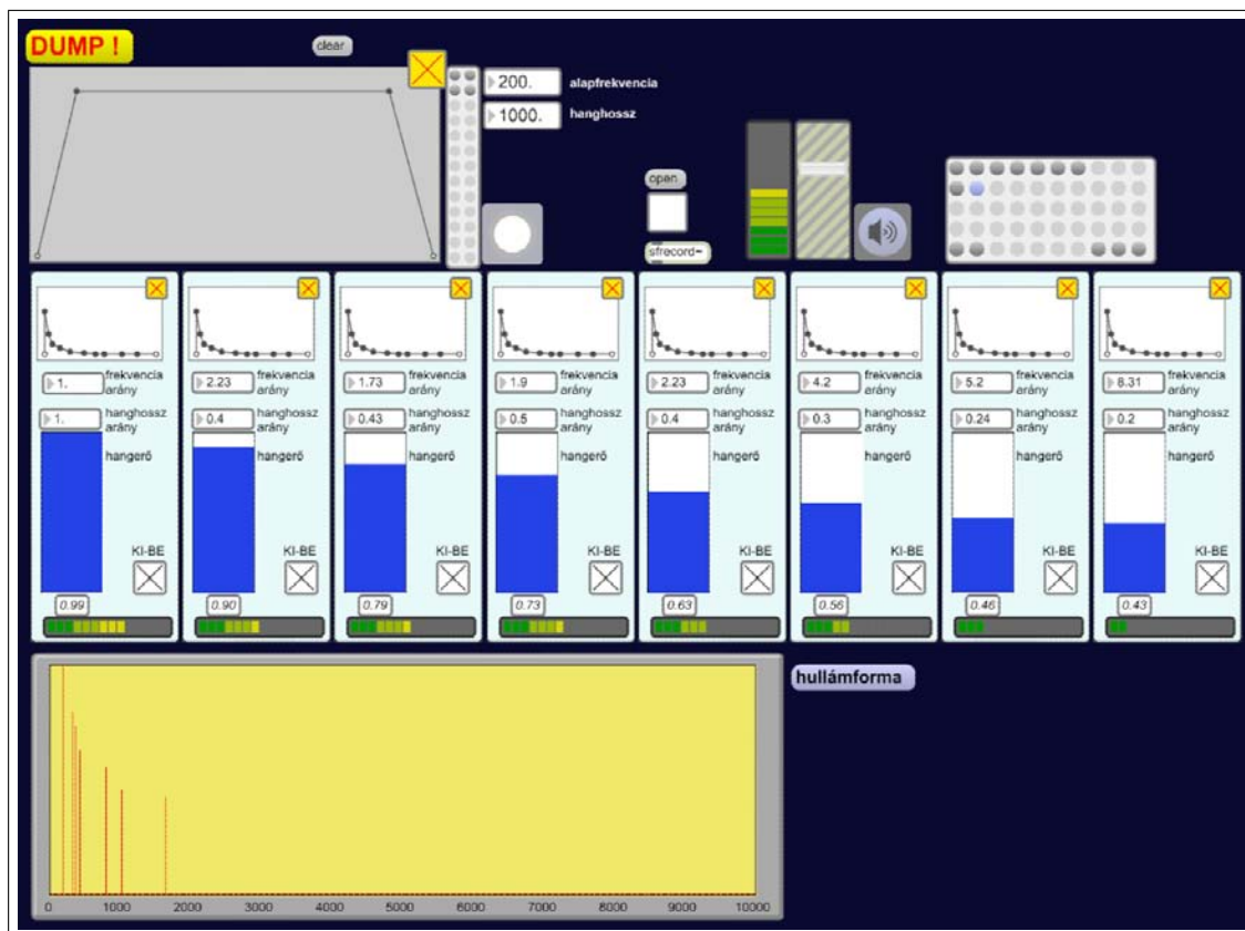
3.3. ábra. Nyolc csatornás additív szintetizátor. A csatornák időtartam-, frekvencia- és amplitúdó-arányai, valamint amplitúdó-burkológörbéi egyedileg szabályozhatóak.
