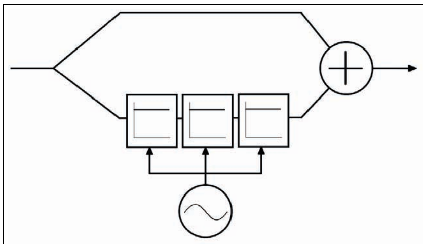
12.2. ábra. Három szűrőt tartalmazó fázistoló folyamatábrája. A szűrők „középfrekvenciáit” (mely jelen esetben azt a frekvenciát jelenti, ami felett a szűrő megfordítja a fázist) egy szinuszos oszcillátor modulálja.
