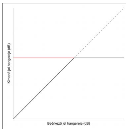
14.2. ábra. Adott határérték fölött levágó limiter karakterisztikája. A 14.1. ábra bal oldalán található karakterisztikával összehasonlítva látható, hogy a limiter valójában egy kompresszor, ahol a \infty:1 tömörítési arány miatt a karakterisztika határérték feletti része teljesen lapos.
