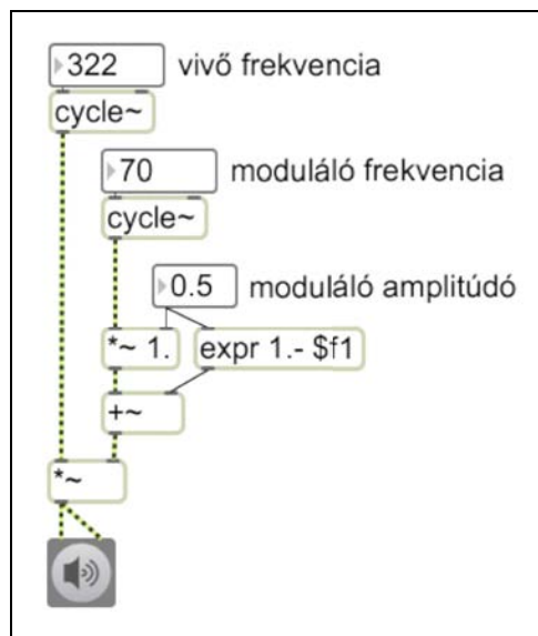
8.4. ábra. Amplitúdó-moduláció Max programnyelven (HApp_08_01 (OSX) (WIN)).
