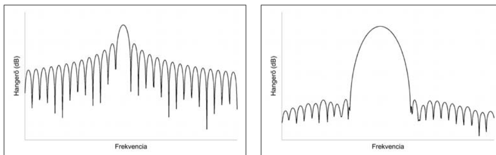
10.2. ábra. Szinuszhullám spektruma négyszögletes (bal) és Blackman–Harris (jobb) ablakfüggvények használatával (a „valódi” spektrum egyetlen frekvenciát tartalmazna, ahogy az az 1.1. ábrán látható). Míg a négyszögletes ablaknak a frekvenciafelbontása, addig a Blackman–Harrisnek a zajszintje kíváló.
