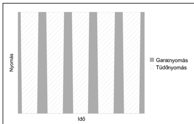
7.3. ábra. A tüdőkből kiáramló levegő, illetve a garaton (hangszálak, hangrés) áthaladó légoszlop nyomásának vázlatos képe az idő függvényében.
