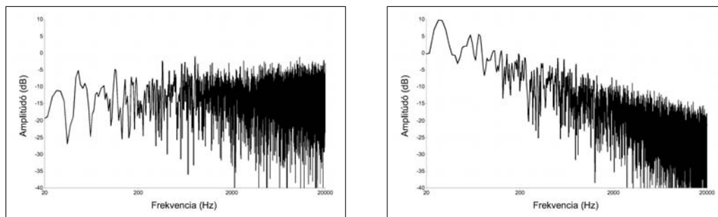
4.1. ábra. Fehérzaj (bal) és rózsazaj (jobb) jellemző spektrumai. Logaritmikus frekvencia-ábrázolás mellett (ekkor az azonos vízszintes távolság azonos hangköznek felel meg) jól látható, hogy míg a frekvenciák amplitúdója fehérzaj esetén gyakorlatilag állandó, a rózsazajban az amplitúdók csökkenő tendenciát követnek (oktávonként 3 dB esést).
