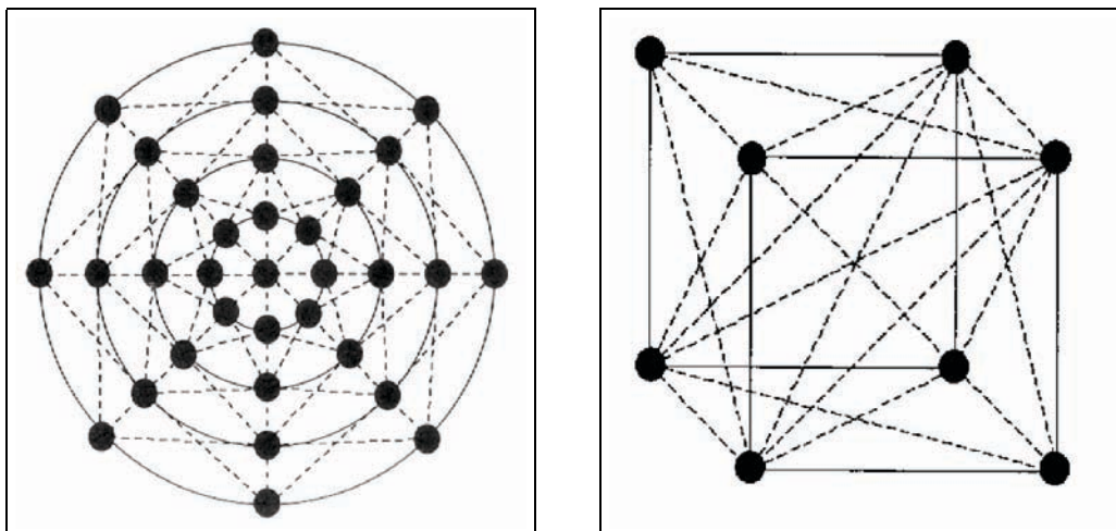
6.2. ábra. Körszimmetrikus (bal) és hasábos (jobb) alrendszerek. A modális szintézis során ilyen alrendszerek kollektív rezgéseit vizsgáljuk.
