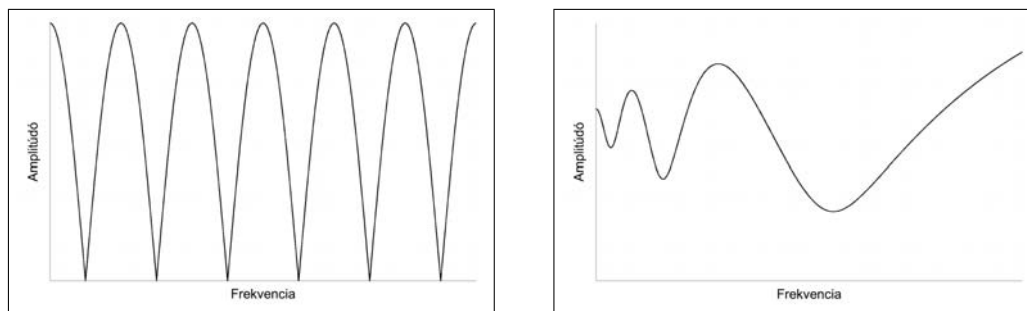
12.3. ábra. A anger (bal) és a fázistoló (jobb) jellemző spektrumai.
