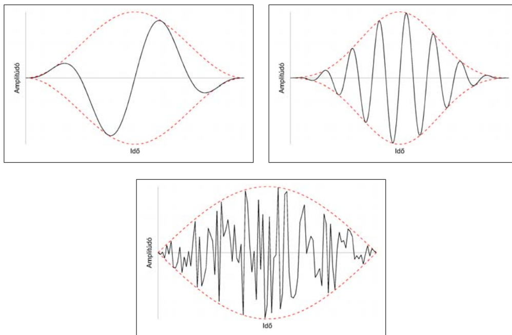
5.1. ábra. Három különböző hangszemcse. A szaggatott vonalak az amplitúdó-burkológörbét mutatják, amiket a szemcsék „kivágásához” használtunk (e burkológörbét a gyakorlatban valamilyen ablakfüggvénynek – lásd a 10. fejezetet – szokás választani). A két felső szemcsét szinuszos hangból generáltuk, a kettő közötti hangszínekülönbség az eltérő belső szerkezetből, pontosabban, az oszcillációk eltérő számából adódik (lásd az 5.1. és az 5.2. hangpéldákat). A lentit szemcsét egy zajforrással hoztuk létre (lásd az 5.3. hangpéldát).
