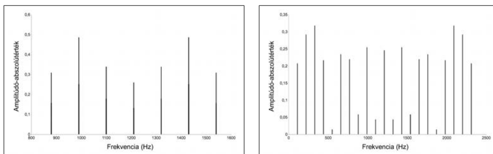
9.5. ábra. A modulációs index hatása a spektrum szélességére. Mindkét esetben f_c = 1210 Hz és f_m = 110 Hz (vagyis H = \frac{1}{11} , a hang harmonikus), azonban míg a bal oldali ábrán I = 3 , a jobb oldalin I = 10 . A két hangot a 9.2. (bal oldali spektrum) és a 9.3. (jobb oldali spektrum) hangpéldák tartalmazzák.
