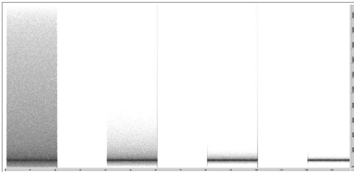
4.3. ábra. Fehérzaj szűrése több lépcsőben. A felhasznált alapszűrő egy sáváteresztő karakterisztikájú, 1 000 Hz középfrekvenciájú, 100 Hz sávszélességű szűrő. Az egyes lépésekben rendre 1, 2, 3 és 4 ilyen szűrőt kapcsolunk össze soros elrendezésben. A szonogram függőleges tengelyén a frekvencia (Hz), vízszintes tengelyén az idő (másodperc) szerepel. Az eredményt a 4.3. hangpélda tartalmazza.
