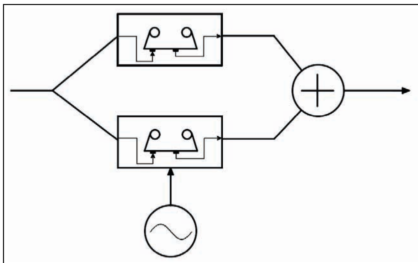
12.1. ábra. Flanger folyamatábrája. A felső késleltető konstans időt késik, az alsó késési idejét egy szinuszos oszcillátor modulálja.
