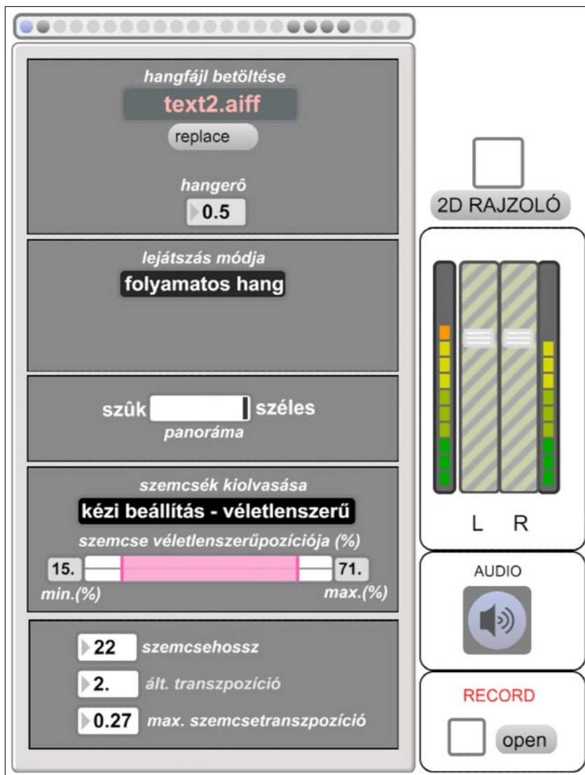
5.2. ábra. Egy granuláris szintetizátor kezelőfelülete. A program a szemcséket egy hang le- ből vágja ki.
