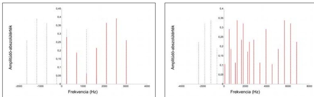
9.8. ábra. Tükröződő spektrumok. A tükrözés előtti állapotot a pontozott fekete spektrum, a tükrözés utáni végeredményt a piros spektrum mutatja. A bal oldali ábrán H = \frac{f_m}{f_c} = \frac{466 \text{ Hz}}{699 \text{ Hz}} = \frac{2}{3} (ebből az alaphang f_0 = 233 \text{ Hz} ) és I = 5 . Mivel \frac{2}{H} = 3 , vá- rako- zása- inknak megfelelően a tükrözött frekvenciák az eredetiekkel átfedésbe ke- rülnek. A jobb oldali ábrán H = \frac{f_m}{f_c} = \frac{574 \text{ Hz}}{2214 \text{ Hz}} = \frac{7}{27} (ebből az alaphang f_0 = 82 \text{ Hz} ) és I = 8 . Mivel \frac{2}{H} = \frac{27}{14} , a tükrözött frekvenciák új komponenseket illesztenek a spektrumba. Mivel f_c \bmod f_m = 492 \text{ Hz} (ami megegyezik f_m - f_0 -al), a kapott hang, habár – matematikai értelemben – harmonikus, nagyon szélesen elhelyezke- dő frekvencia-párokat tartalmaz, így nem alakul ki igazi hangmagasság-érzet. A két hangot a 9.6. (bal) és a 9.7. (jobb) hangpéldák tartalmazzák.
