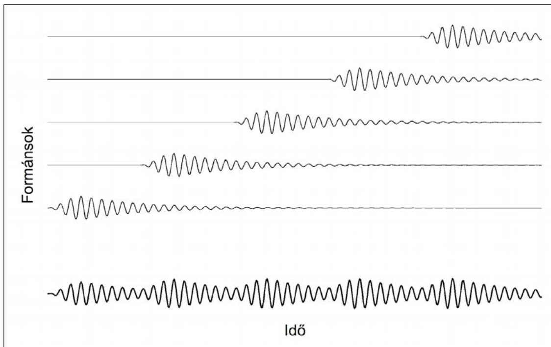
7.10. ábra. A FOF-szintézis folyamata. Az alapfrekvencia által diktált pillanatokban egy-egy új hullámot generálunk (ezeket mutatják az egymás fölé helyezett formánshullámok), az így kapott hullámformákat pedig összeadjuk. Amint az ábrán is látható, általában az egyes alap-hullámformák később érnek véget, mint amikor a következő visszajátszás kezdődik, így „többszörös kiolvasással” kell élnünk.
