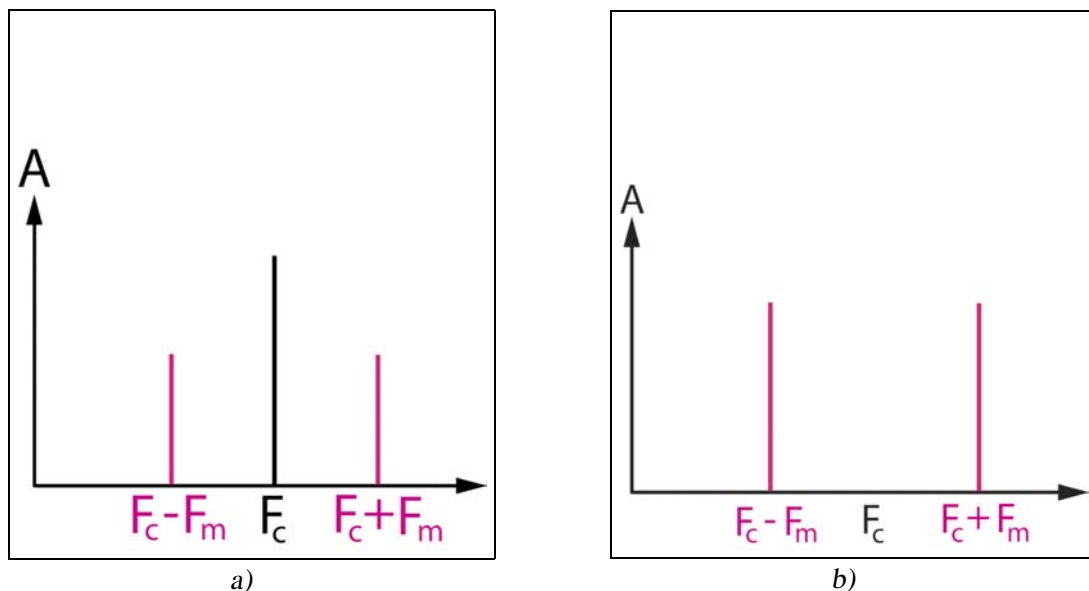
8.2. ábra. Az amplitúdó- (a) és ringmoduláció (b) spektruma.
