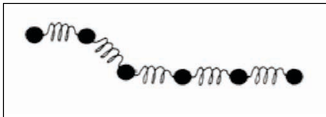
6.1. ábra. Tömegpont-rugó modell. Az ábrán a bal oldali tömegpont kitérített állapotban van, a modellezés során lépésenként modellezzük, hogy e kezdeti kitérés hatására hogyan mozog a teljes rendszer.
