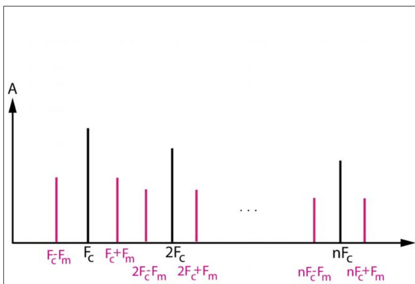
8.3. ábra. Amplitúdó-moduláció komplex vivőhullámmal.
