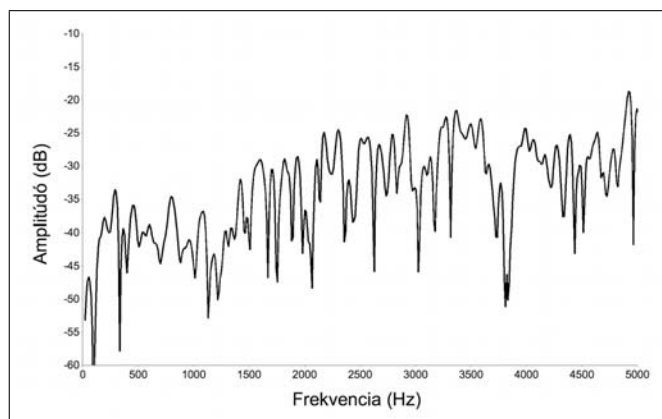
7.2. ábra. Egy „sz” mássalhangzó spektrumának alsó tartománya. Láthatjuk, hogy ez a spektrum nem jellemezhető pusztán néhány csúcs megadásával.
