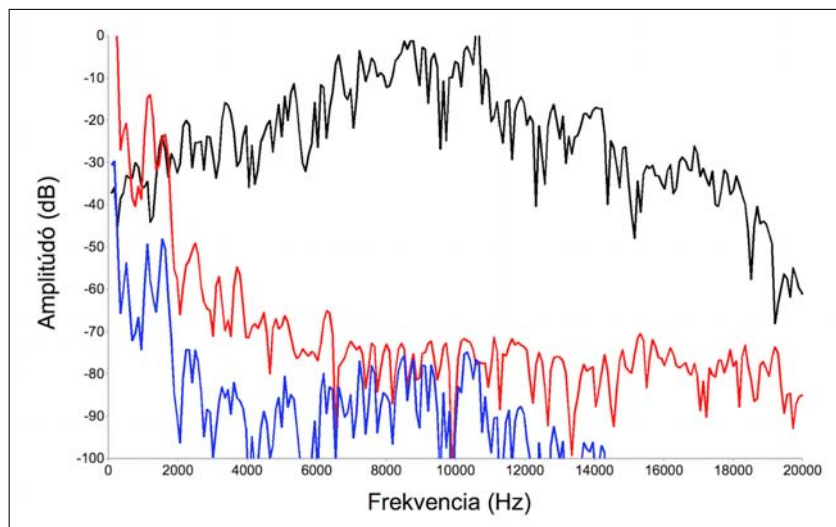
11.4. ábra. Keresztzszintézisben részt vevő spektrumok. A fekete spektrum a vivőjelhez tartozik (zajszerű forrás), a piros pedig a moduláló jel (hangszerhang). A végeredményt a kék spektrum mutatja.
