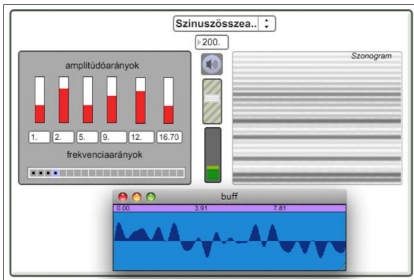
2.5. ábra. Hullámforma létrehozása szinuszok összeadásával. Figyeljük meg, hogy a nem-egész arányok következtében a kapott hullámforma a periódus végén megszakad, emiatt a hangban lesz egy kattánás, torzulás. A szonogramban így sokkal több szinusz jelenik meg, mint amennyit az összeadáshoz felhasználtunk.
