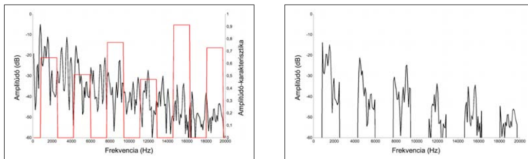
11.2. ábra. Többsávós spektrális szűrő. Bal oldalon a forrás spektruma és a szűrő-karakterisztika (piros vonal), jobb oldalon a szűrt spektrum látható. A 11.9. hangpélda többsávós szűrővel szűrt fehérzajt tartalmaz.
