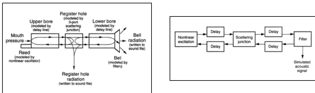
6.4. ábra. Egy fúvós hangszer (klarinét) nagyon egyszerű modellje. A fúvókának egy zajszerű gerjesztés, a csőnek különböző késleltetők, míg a hanglyuknak és a tölcsérnek egy keverő és egy szűrő felel meg.
