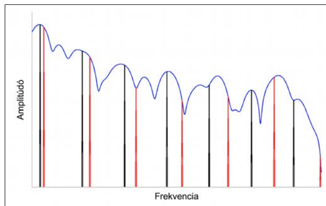
11.1. ábra. Transzpozíció az eredeti spektrális burkológörbe megtartásával. Az eredeti spektrumot a fekete, a spektrális burkológörbét a kék, az új spektrumot a piros vonalak jelzik. Figyeljük meg, hogy (mivel transzponáláskor a frekvenciák aránya az, ami változatlanul marad) a távolság az új és az eredeti komponensek között a frekvencia növekedésével arányosan nő.
