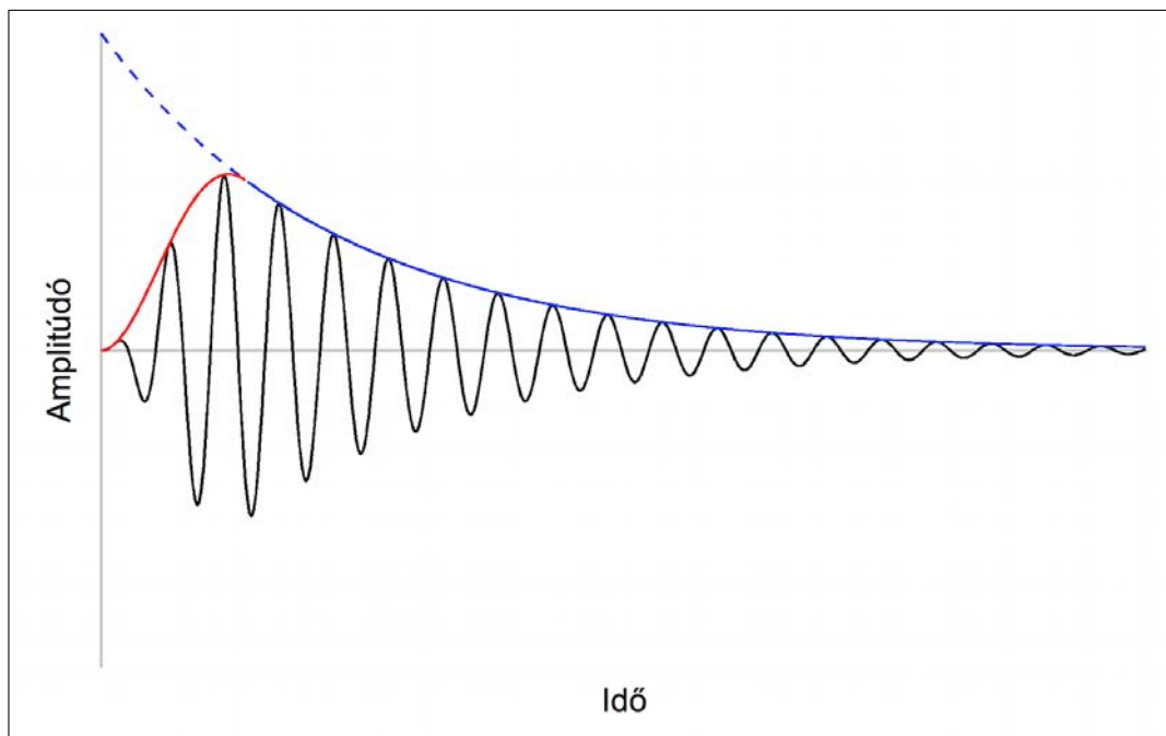
7.9. ábra. A (7.1) egyenlet által leírt függvény. A kék vonal az \alpha által megszabott exponenciális esést, a piros vonal a \beta által szabályozott koszinuszos indítást mutatja. A két görbe t = \frac{\pi}{\beta} -nál találkozik. A végeredményt (a modulált szinuszhullámot) a fekete jel ábrázolja.
