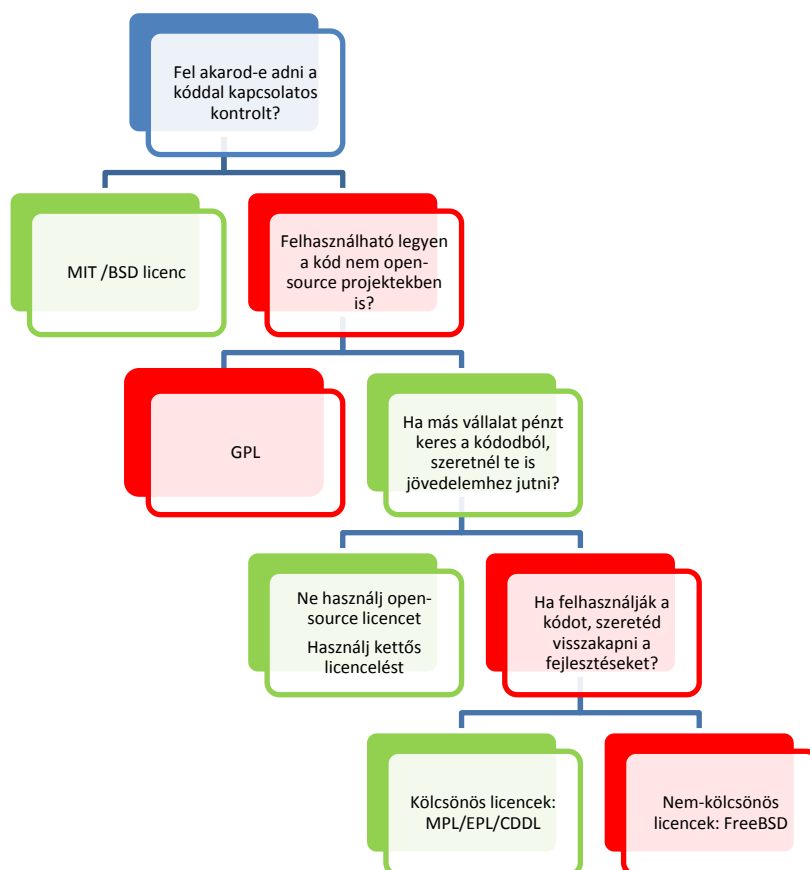
4.1. ábra: Licencválasztást segítő folyamatábra. Zöld doboz, ha a korábban feltett kérdésre igen, piros, ha nem volt a válaszod
