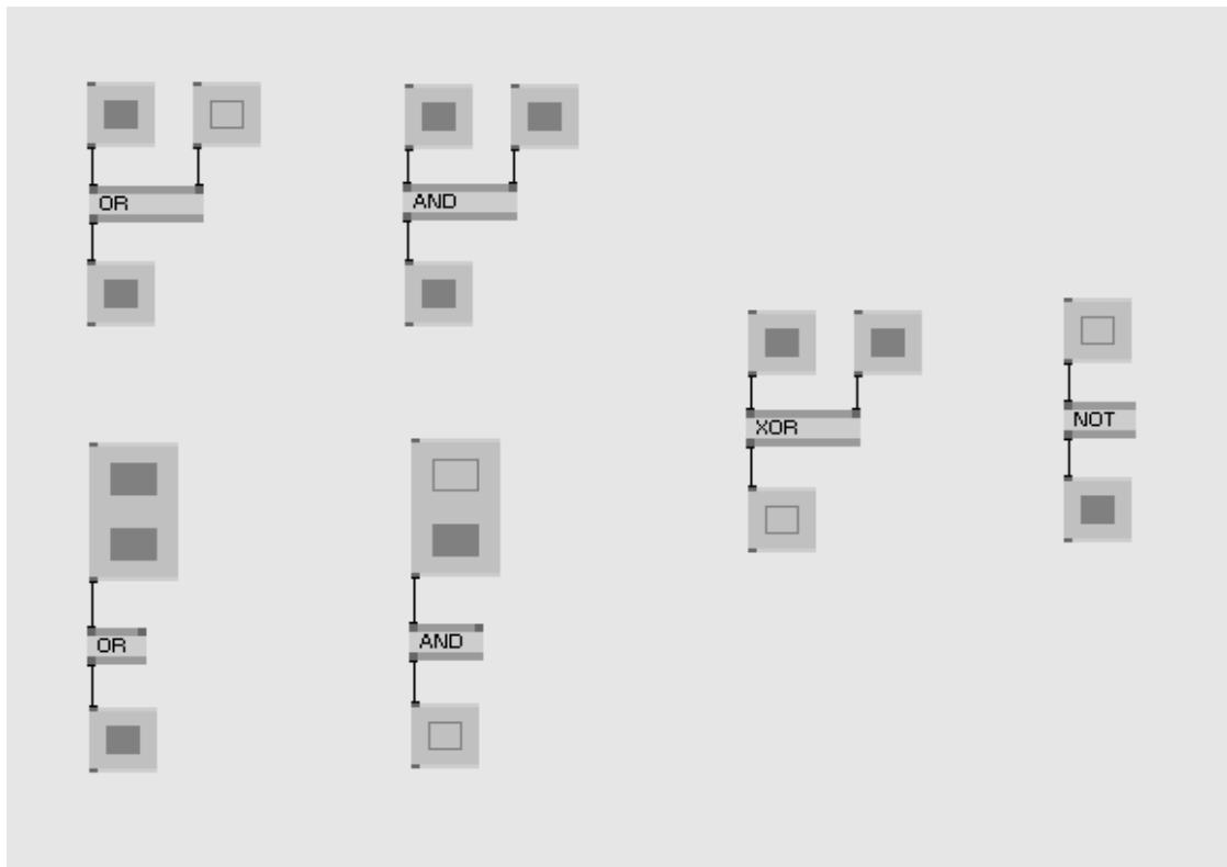
4.3. ábra: Logikai kapuk használata
