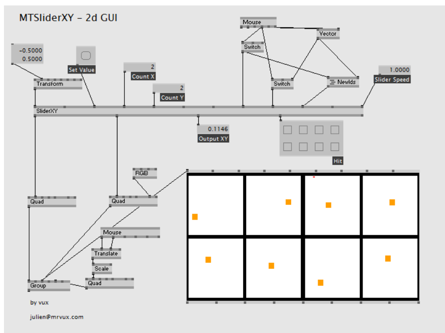
15.4. ábra: XY Slider Gui Multitouch
