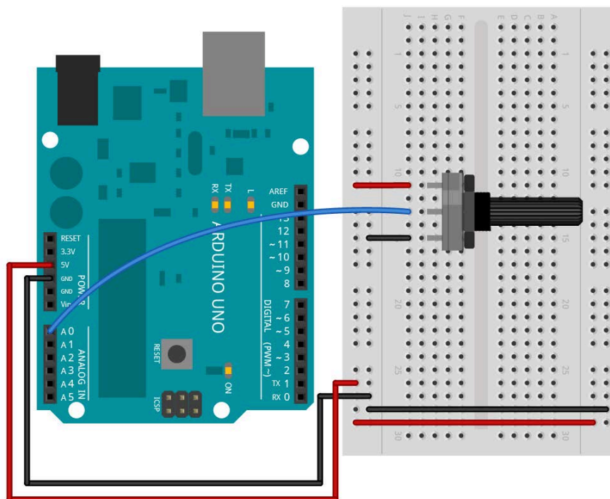
13.32. ábra: Arduino potméter bekötése
