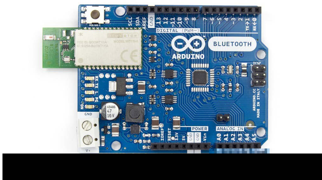
13.3. ábra: Bluetooth Arduino
