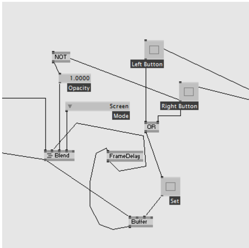
9.3. ábra: Blend és a Buffer bekötése
