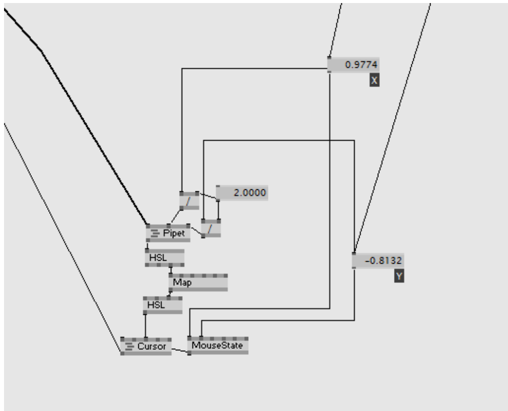
9.4. ábra: Cursor és a Pipet bekötése
