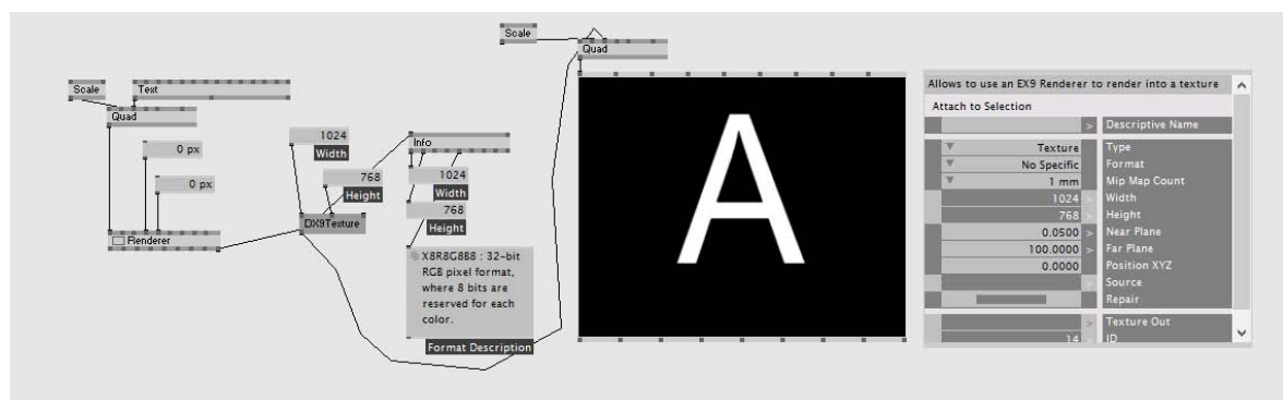
9.9. ábra: Felbontás beállítása DX9Texture-ben
