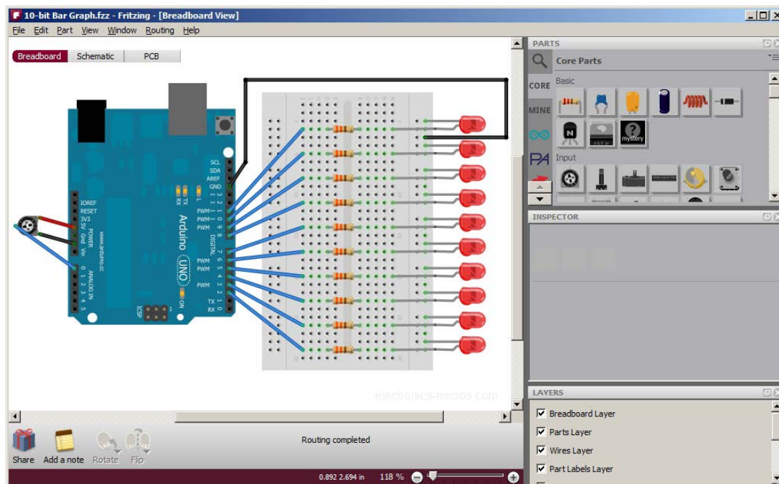
13.25. ábra: Arduino Fritz
