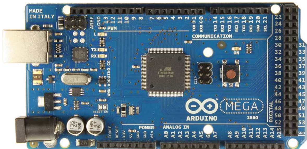
13.5. ábra: Arduino Mega
