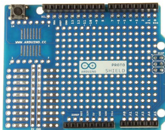
13.17. ábra: Proto shield
