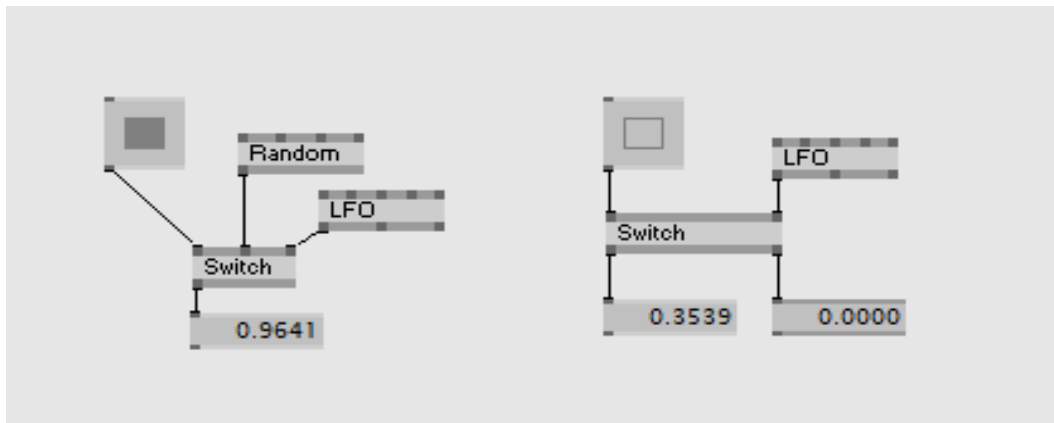
4.5 ábra: Bemenet- és kimenetkapcsolók
