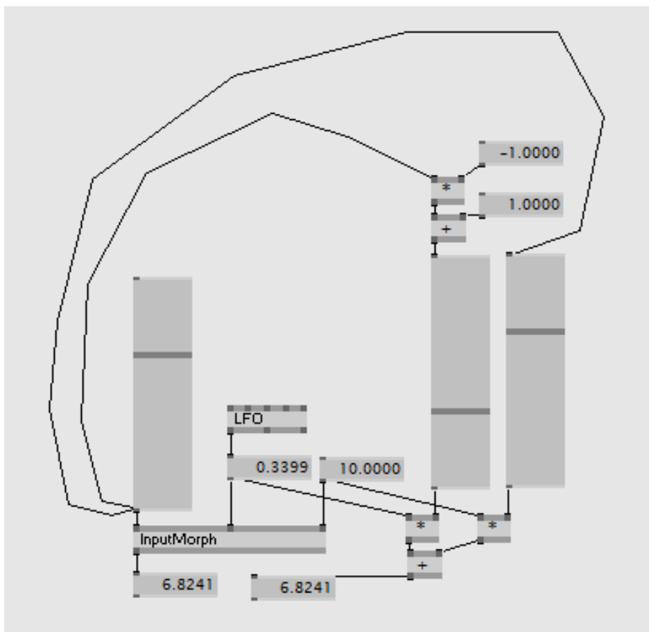
4.7. ábra: Az InputMorph
