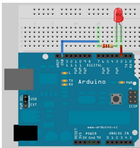
13.30. ábra: Arduino Led bekötése
