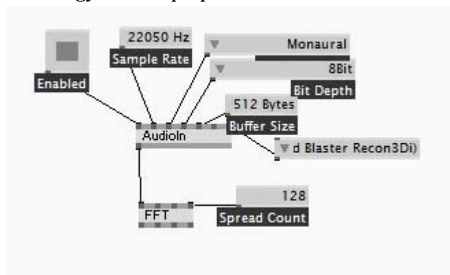
10.4. ábra: AudioIn és az FFT
