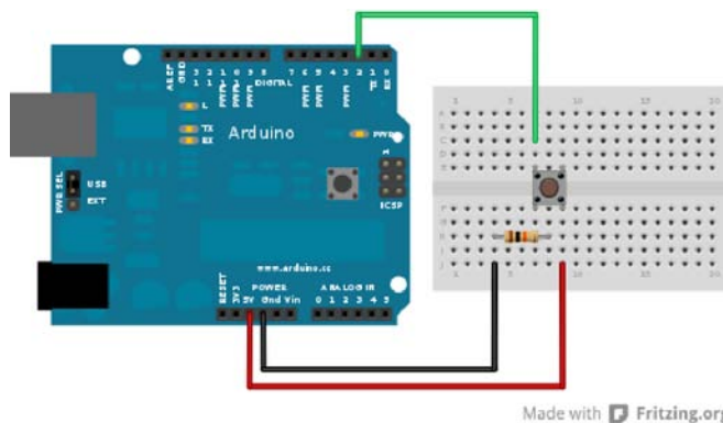
13.31. ábra: Arduino kapcsoló bekötése
