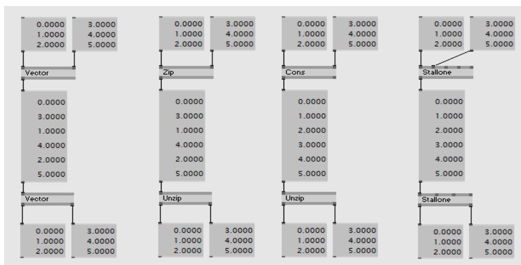
4.12. ábra: A Vector, Zip, Cons és a Stallone
