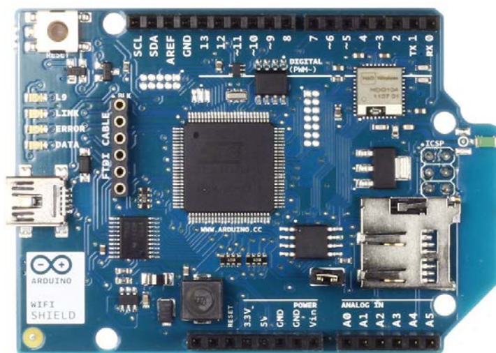
13.12. ábra: Wifi shield
