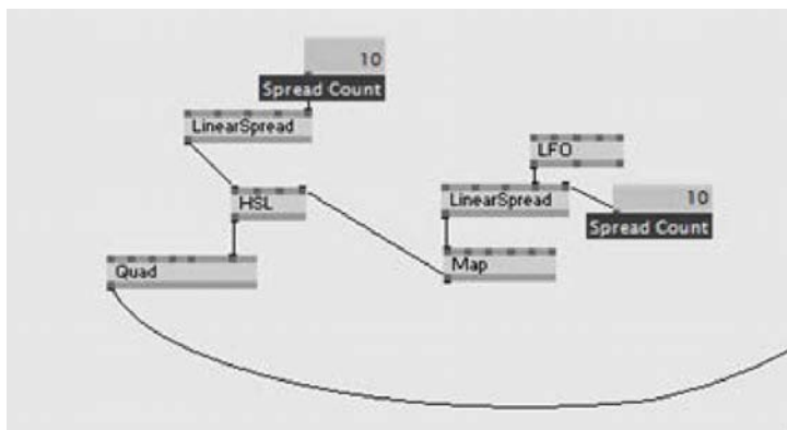
6.4. ábra: HSL LinearSpread
