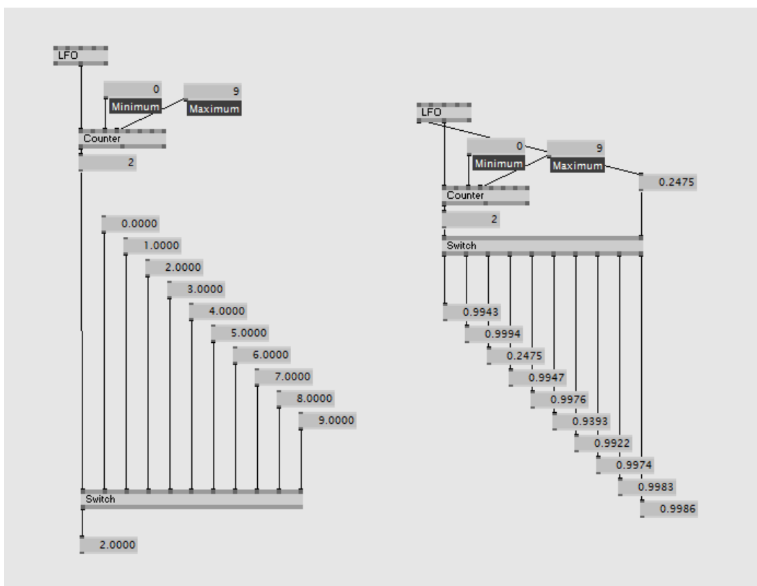
4.6. ábra: Kapcsolók több ki-, ill. bemenettel
