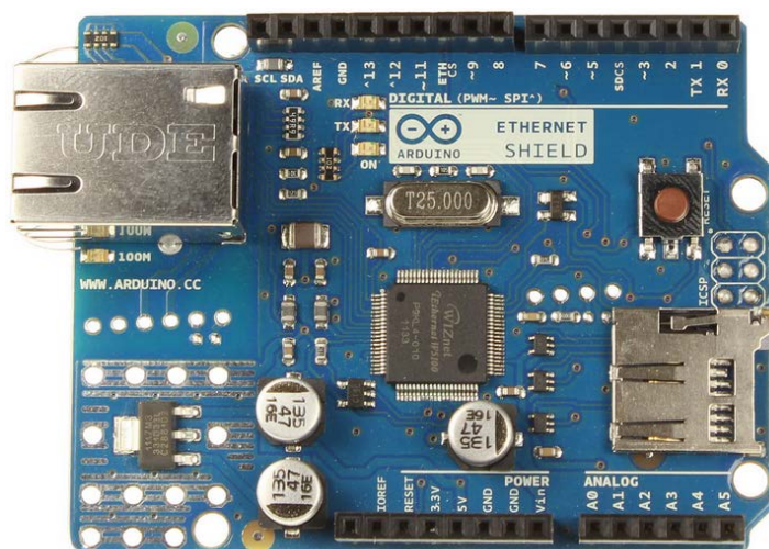
13.16. ábra: Ethernet shield
