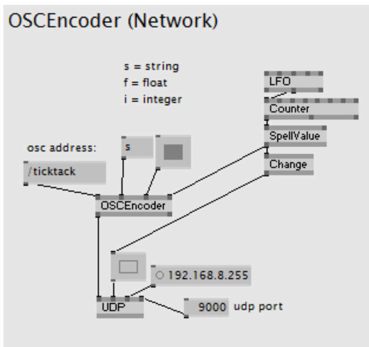
14.4. ábra: Udp küldő
