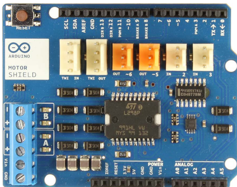
13.20. ábra: Motor shield
