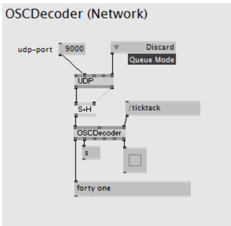
14.3. ábra: Osc fogadó
