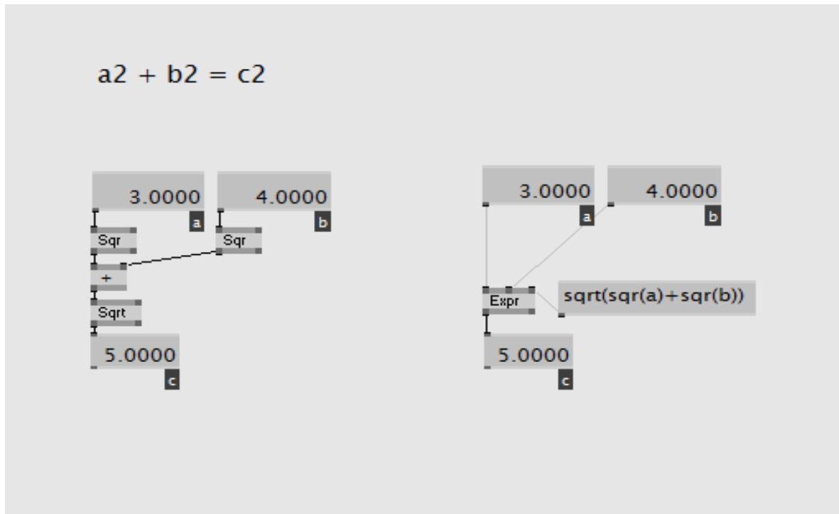
4.2. ábra: Komplexebb matematikai műveletek
