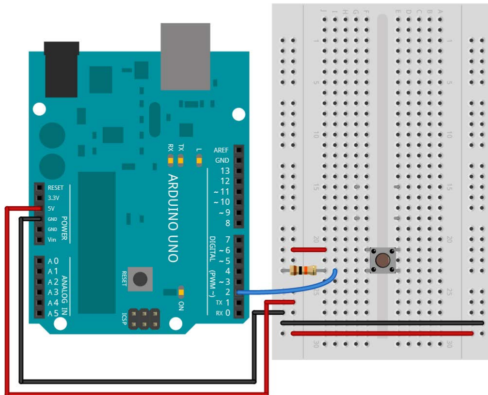
13.26. ábra: Arduino bekötési minta
