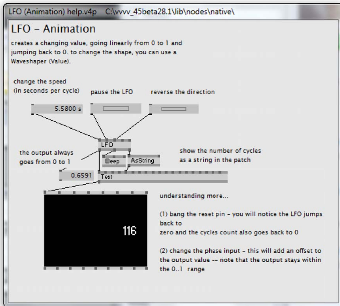
2.11. ábra: Lfo segédfájl
