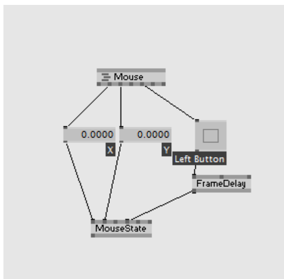
10.6. ábra: Mouse és MouseState TagPointhoz
