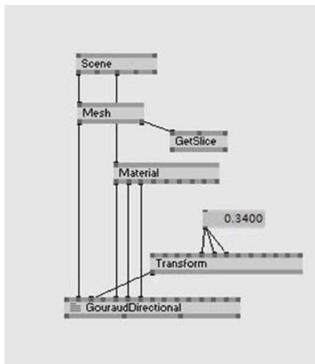
7.1. ábra: A Scene betöltő modul
