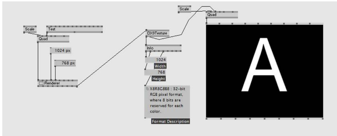
9.8. ábra: Felbontásbeállítással eltüntetett Render
