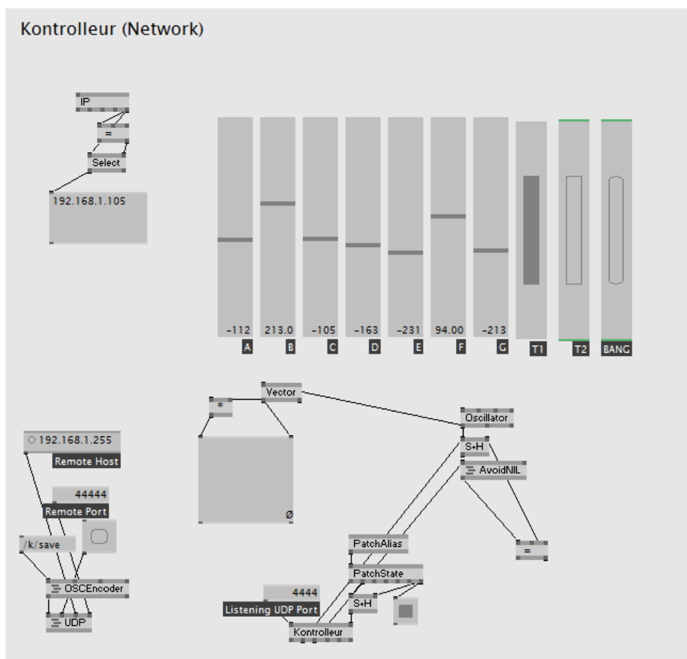
12.12. ábra: Kontrolleur patch
