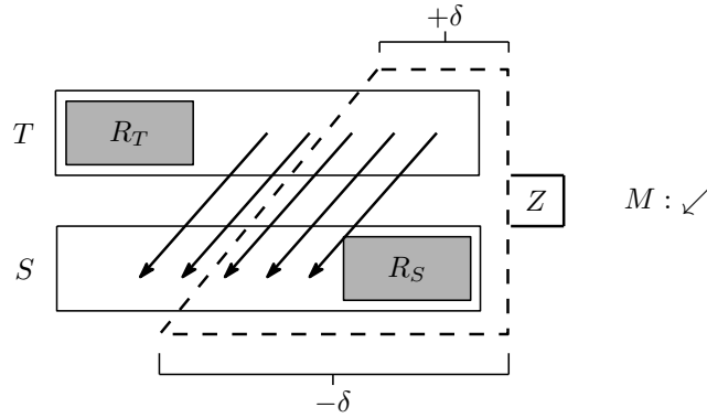
1.2. ábra. A \pi változtatása a magyar módszer egy lépésében
