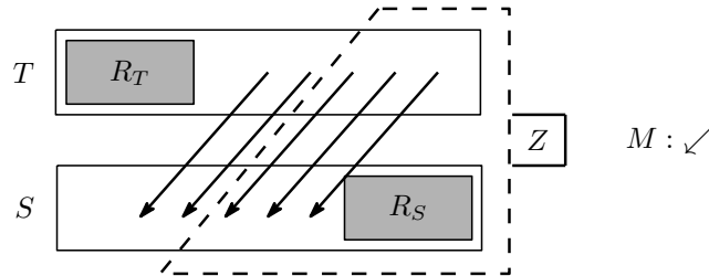
1.1. ábra. A König-tétel bizonyításának illusztrálása
