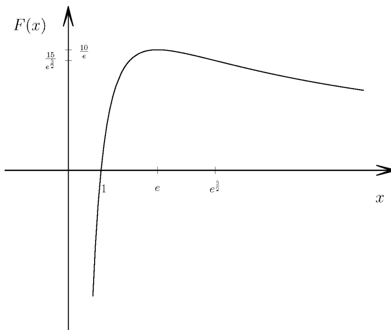
8.9. ábra. Az F(x) := \frac{10 \ln(x)}{x} , D(F) := \mathbb{R}^+ függvény grafikonja
